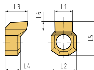
figura 1 - INSERTO PER SEDI DI CHIAVETTE (IBM) picture 1 - INSERT FOR INTERNAL KEYWAY (IBM)
